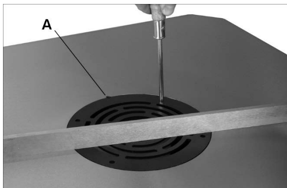
Рис. 6: установка вставки стола
